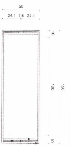
VISTA SUPERIOR
