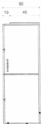
CORTE PARTE INFERIOR DO MÓVEL
