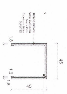
CORTE BB
