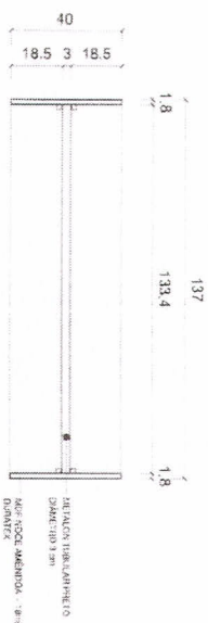
CORTE A
